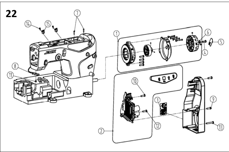
二十二、DI部件专用件(DI specific parts)
