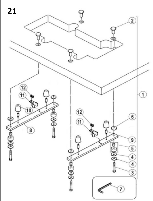
二十一、油盘托板部件(Oil plate assemblies)
