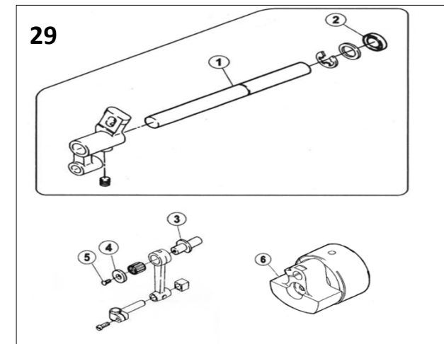
二十九、 21、22专用部件 (21、22 specific parts)
