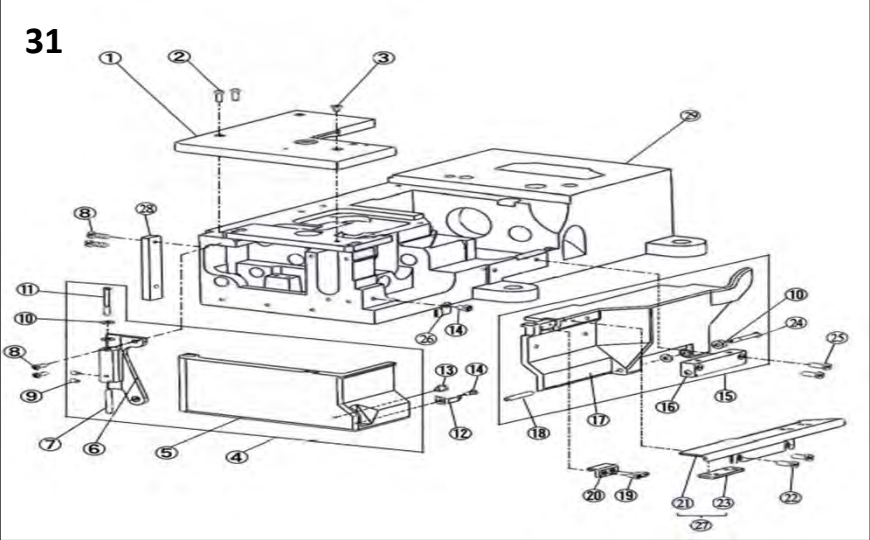
三十一、 W4N专用部件 (W4N specific parts)
