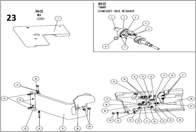
二十五、05专用部件(05 specific parts)
