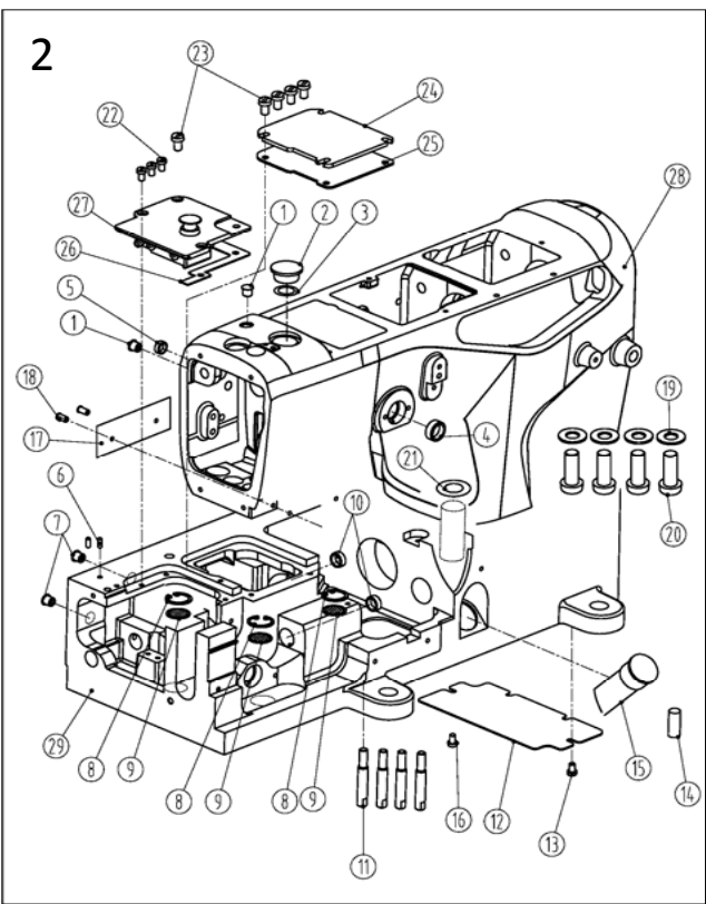
二、车架部件 (Frame assemblies)
