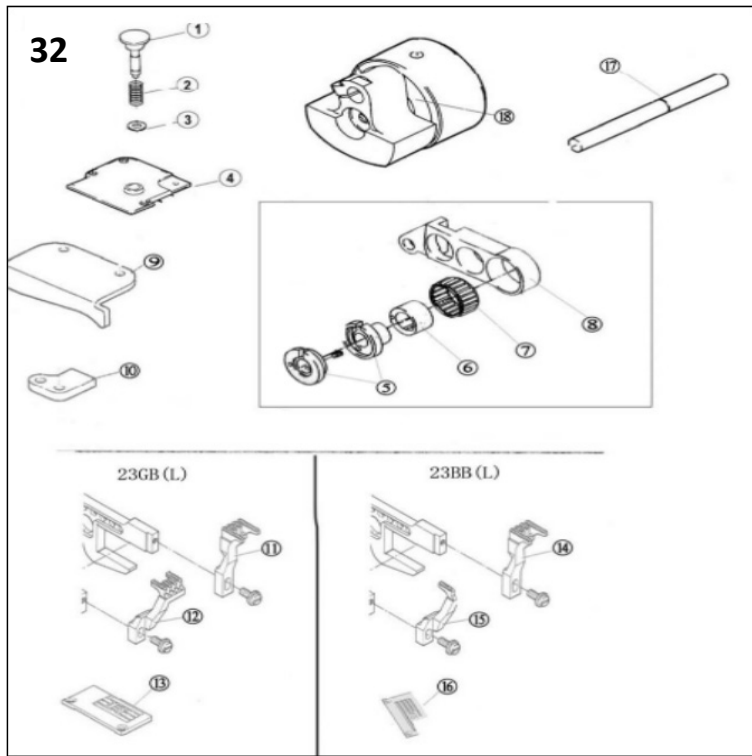
三十二、23专用部件 (23 specific parts)
